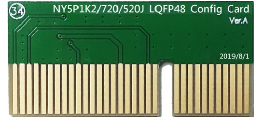
NY5P1K2/720/520J LQFP48 轉卡 (Config Card)
