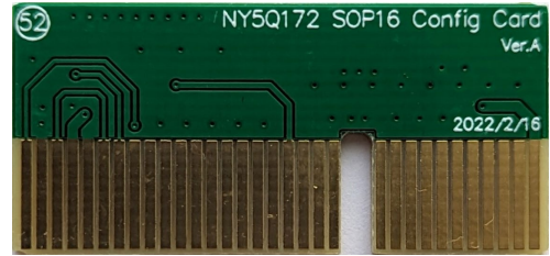
NY5Q172 SOP16 轉卡 (Config Card)
