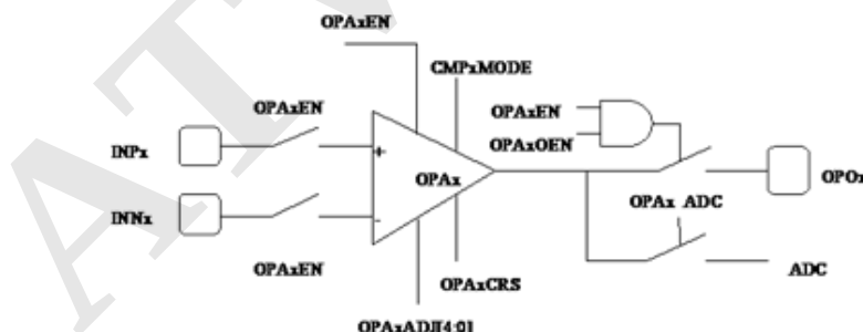
Figure 53 OPAx BLOCK(OPAxOEN SW->OPAxEN & OPAxOEN)
